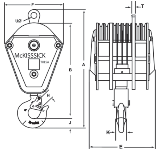
388 – OCTUPLE
